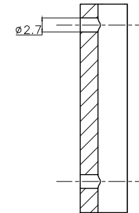
剖面 A-A
